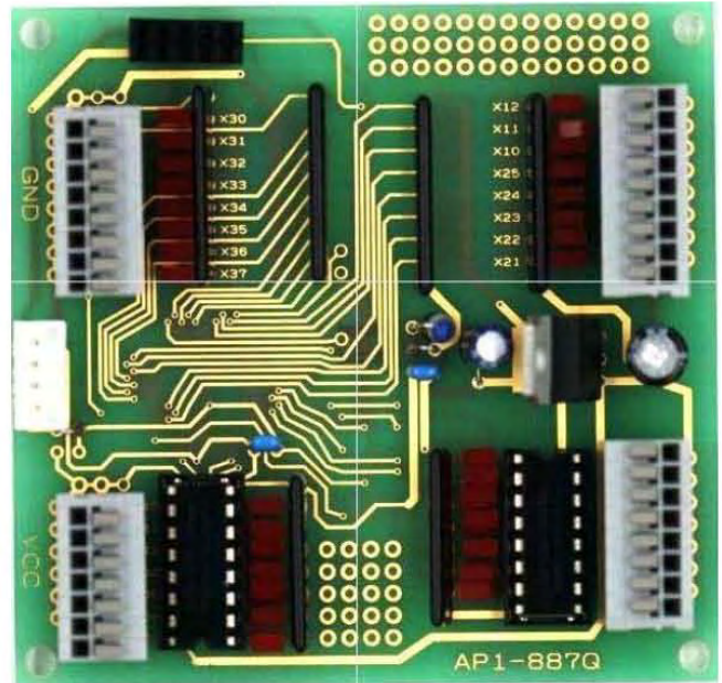
Vcc電源電圧変更及び端子台追加例
